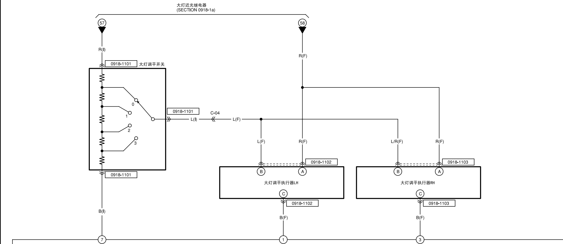
0918-1101 大灯调平开关 (I)
